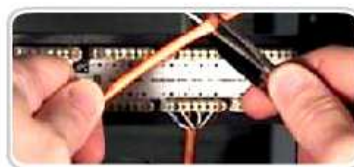
Bloque de inserción a presión 110
