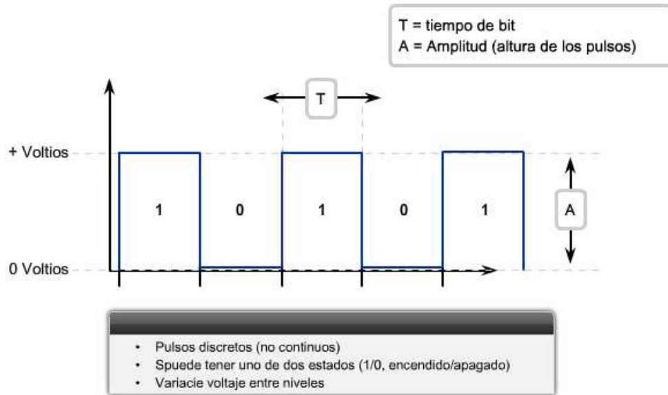
Bits de señalización para la transmisión Sin retorno a cero (NRZ)
